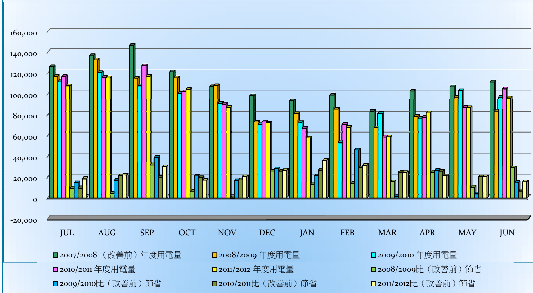
250KVA用戶 2007年七月導入能源管理系統之每月耗電量比較分析
